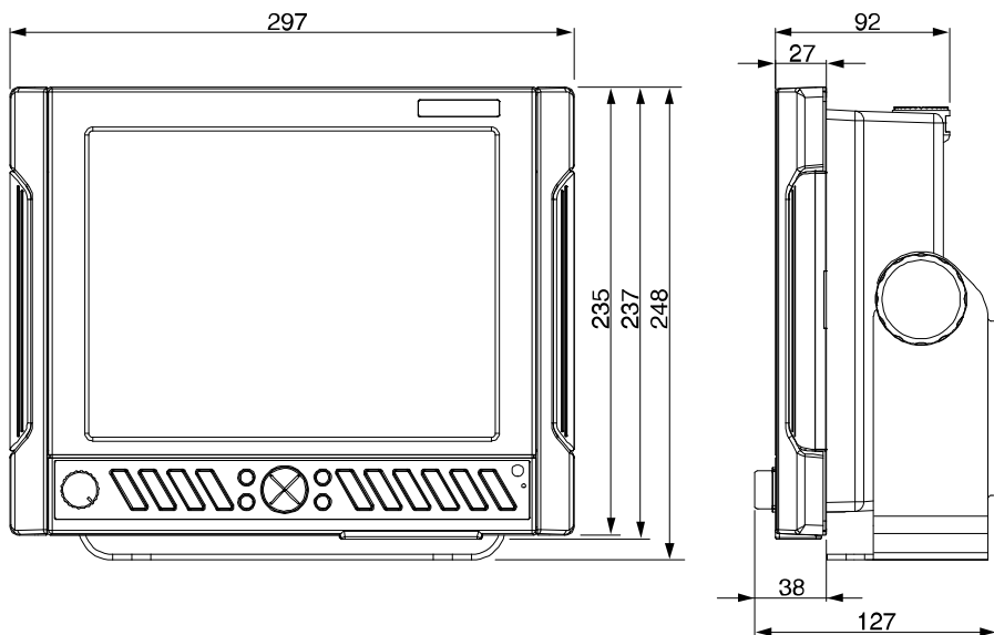
<本体寸法図>
