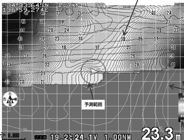
[デブスマッピング®機能で作図中の表示例]
